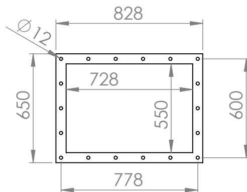
Outlet
